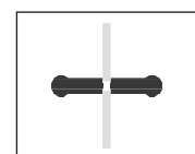
06: Glastür 8 – 14 mm Bohrdurchmesser 13 mm
